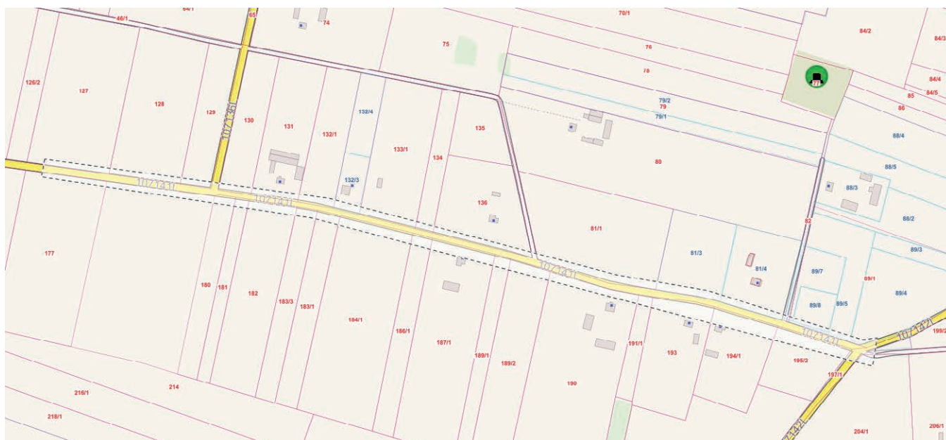
lokalizacja przebudowywanego odcinka DG 107141L w Kiełczewicach Maryjskich
